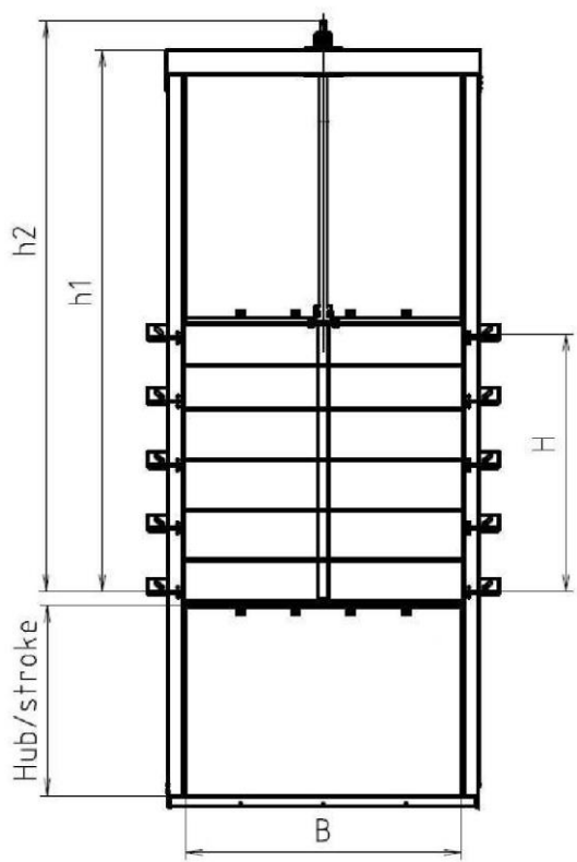
Versiunea cu o tijă
