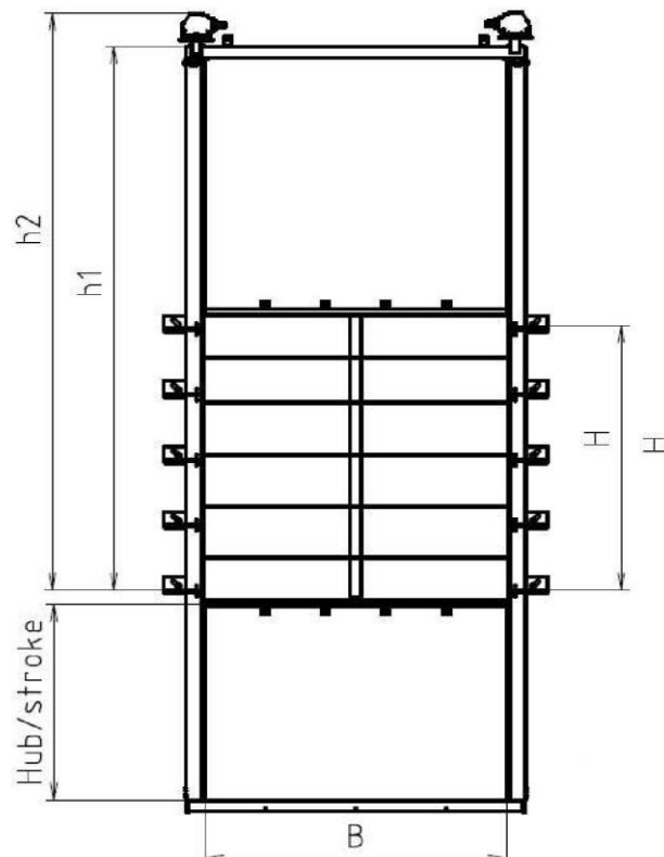
Versiunea cu două tije
